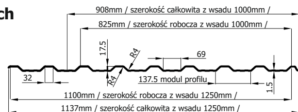
elewacja
