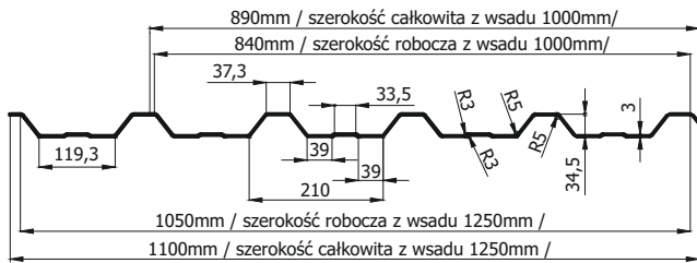
dach
